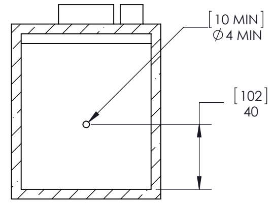
SECTION D-D
